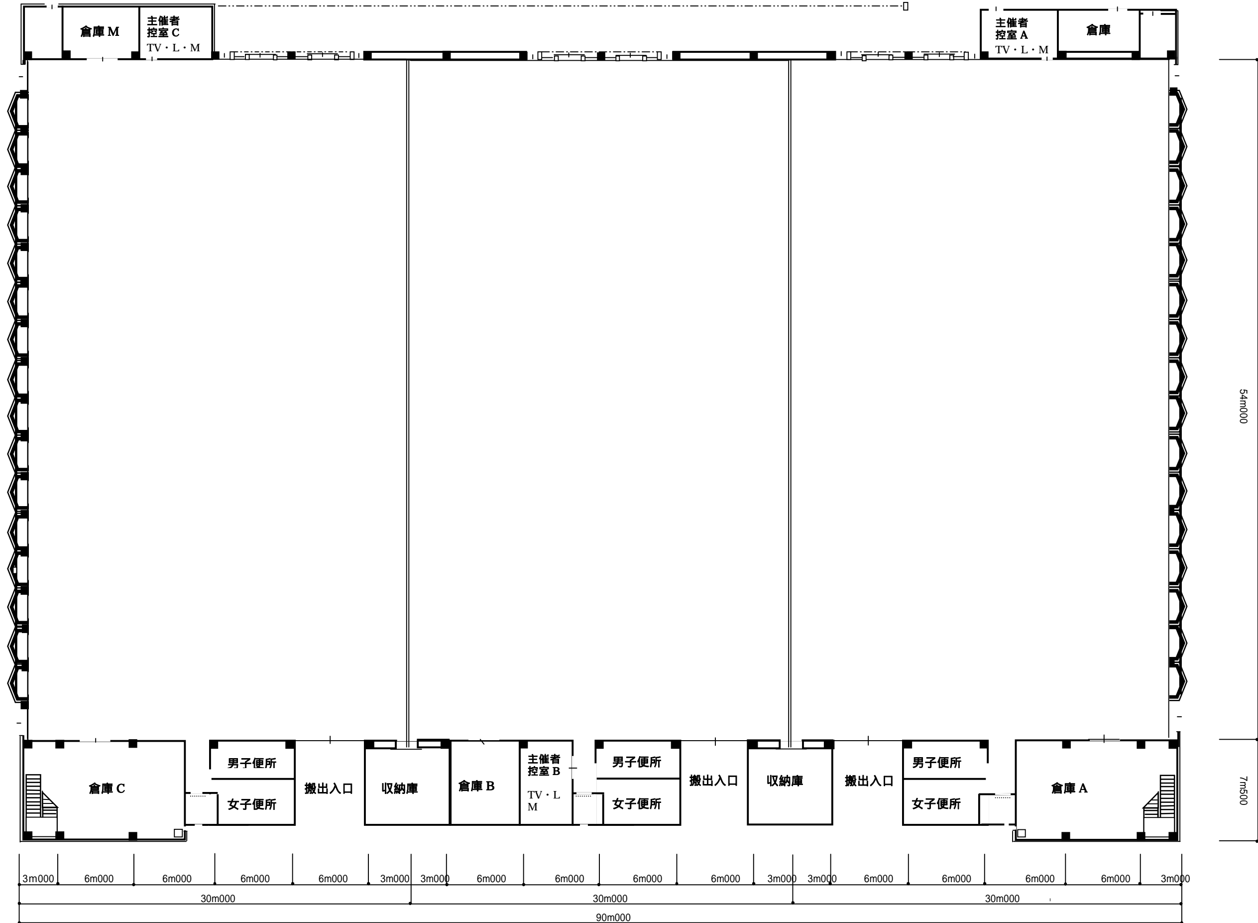
展示ホール 1階平面図 S=1/300
